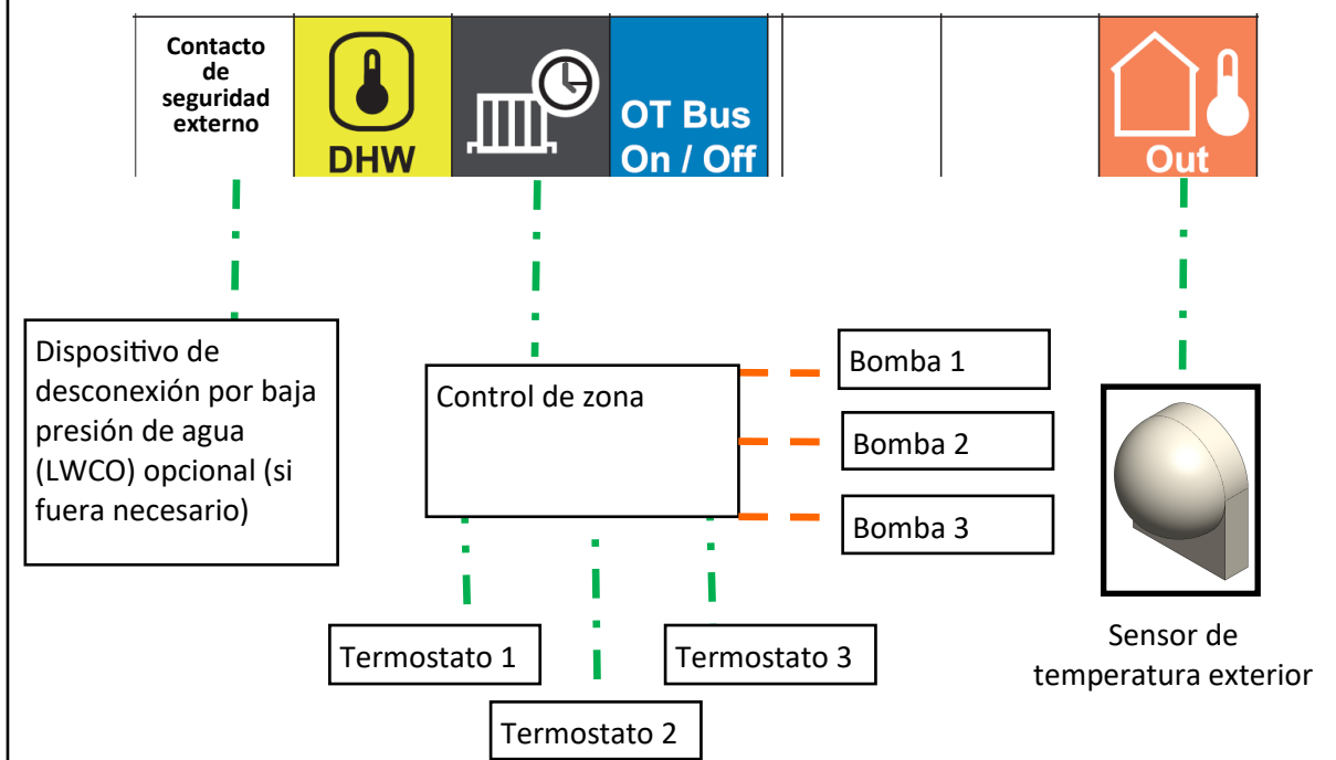
Cableado de la tarjeta de circuito impreso para el ejemplo de aplicación
