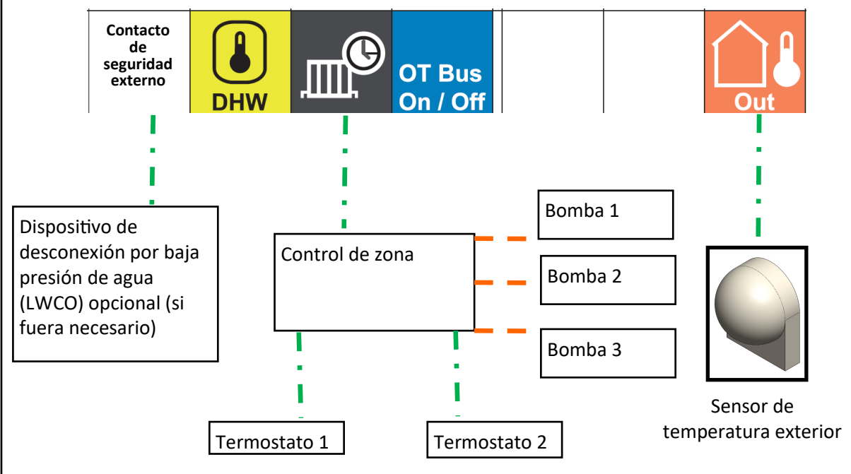
Cableado de la tarjeta de circuito impreso para el ejemplo de aplicación
