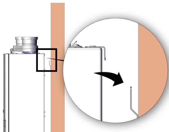
Plantilla de montaje de la caldera
