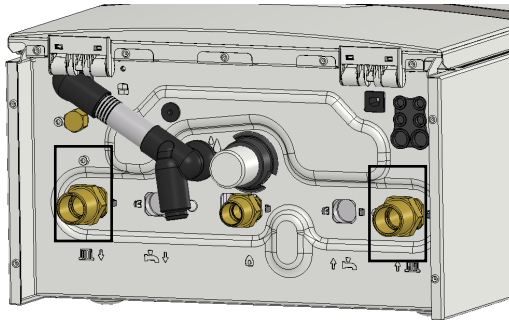
Conexión de suministro y retorno de calefacción
