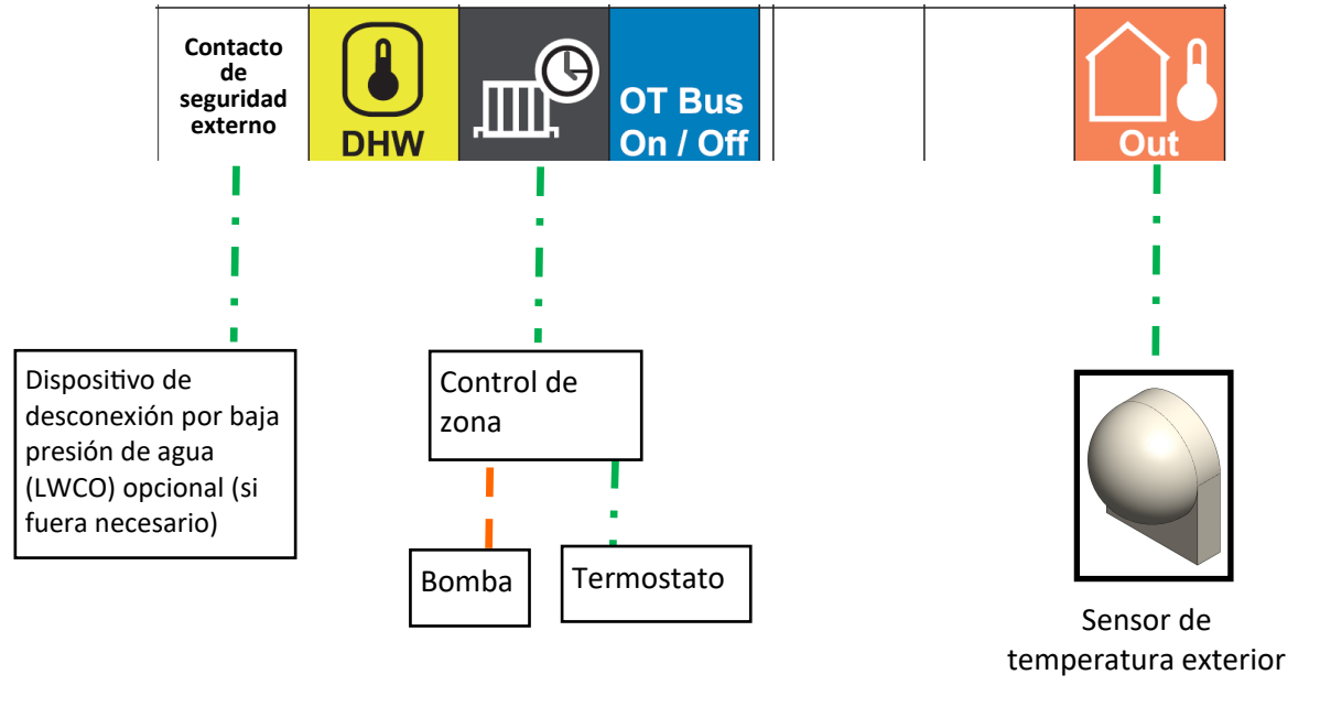
Cableado de la tarjeta de circuito impreso para el ejemplo de aplicación anterior
