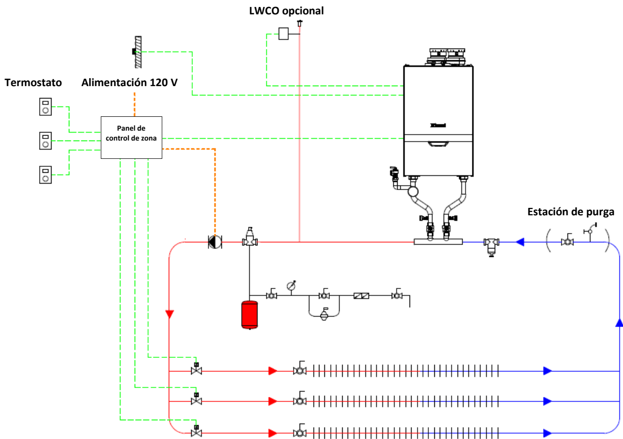
Cableado de la tarjeta de circuito impreso para el ejemplo de aplicación
