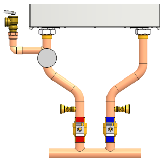
Calentador con juego de calefacción primario-secundario
