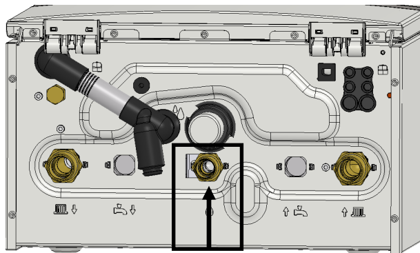
Conexión de gas MNPT 3/4 pulg.
