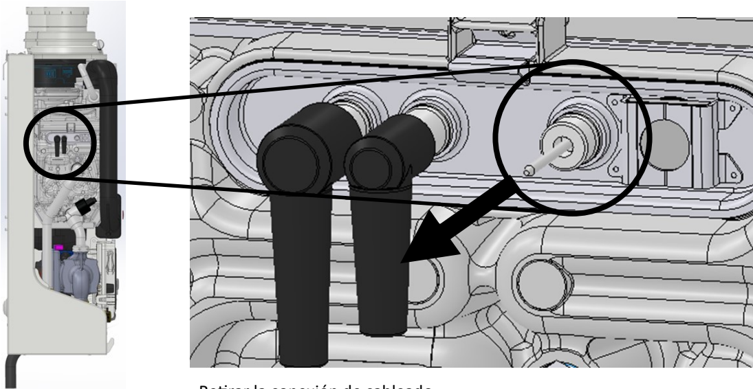
Lado izquierdo de la caldera
